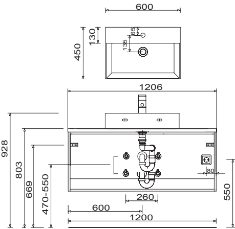
WTM 4806 + APA 5012 66 + WUA 3412 TG
