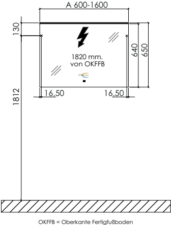
Elektroanschlüsse für Flächenspiegel FSB 41xx 01
