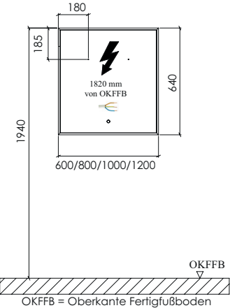
Elektroanschlüsse für Flächenspiegel FSB 45xx 07
