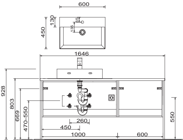
WTM 4806 + APA 5164 66 + WUA SW16 01/03 L
