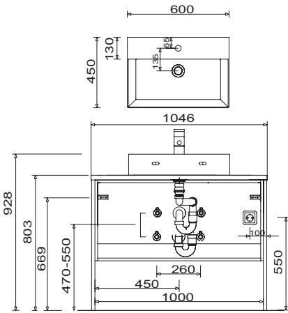
WTM 4806 + APA 5104 66 + WUA SW10
