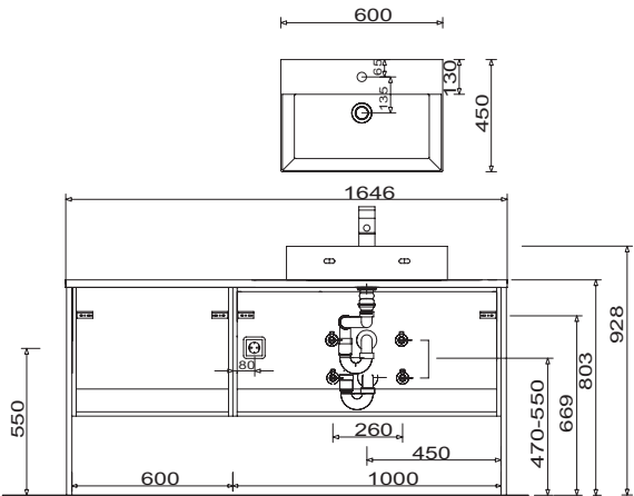
WTM 4806 + APA 5164 66 + WUA SW16 01/03 R
