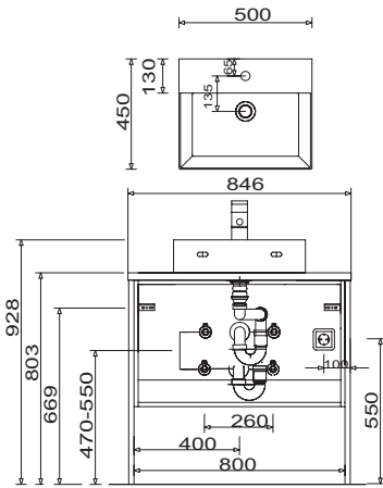
WTM 4805 + APA 5084 66 + WUA SW80
