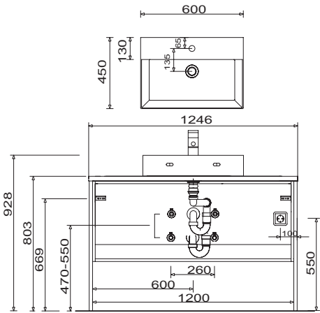
WTM 4806 + APA 5124 66 + WUA SW12
