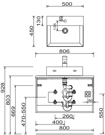
WTM 4805 + APA 5080 66 + WUA 3480 TG
