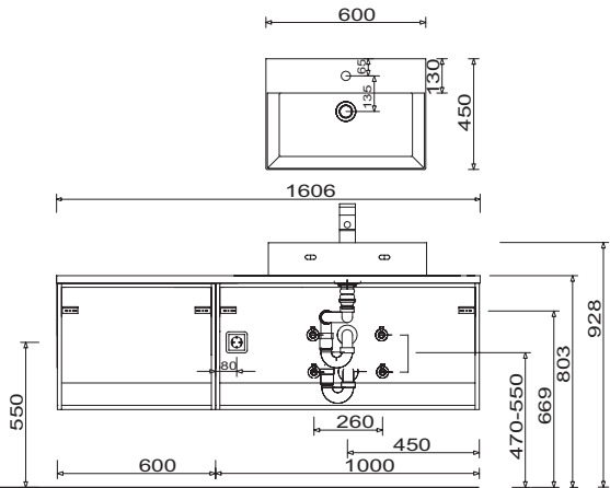
WTM 4806 + APA 5016 66 + WUA SW16 02 R
